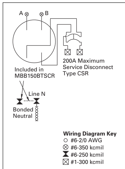
Figure 30. Catalog Numbers – MBB150BTSC, MBB150BTSCR, MBB200BTSCR and MBB200BTSC
