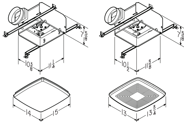
MODÈLES QTXE080, QTXE110, QTXE1102
